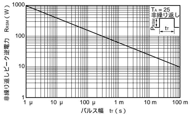
図7 サージ逆電力定格
